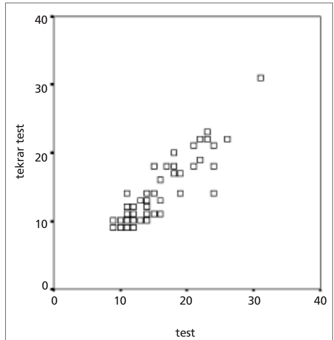
Şekil 1. Test-tekrar test sonuçları arasındaki doğrusal ilişki; r = 0.88, p < 0.001
