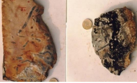
Şekil 17: Gogodere mahallesi civarında tespit edilen Planolites 'e ait iz fosil örnekleri.
