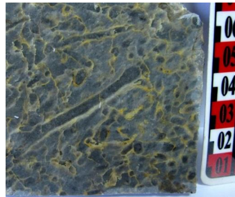
Şekil 20: Gogodere civarında tespit edilen Planolites 'e ait fosilli kayaç örneğinin kesilerek parlatılmış yüzeyi.
