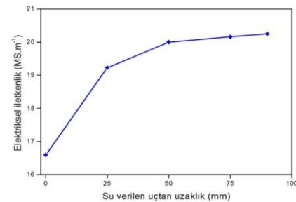
Şekil 4: Su verilen uçtan uzaklaştıkça numunedeki elektriksel iletkenlik değişimi.
