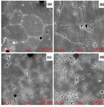
Şekil 5: 480 °C/3h +20 °C su ile soğutma +120 °C/24h yaşlandırma işlemleri uygulanmış numunenin su verilen uçtan farklı mesafelerdeki SEM görüntüleri (a): 5 mm, (b): 25 mm, (c): 50 mm, (d): 75 mm.
