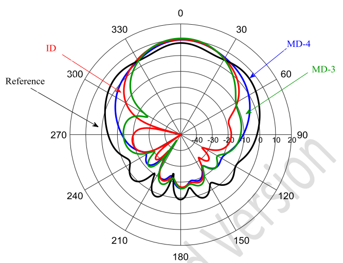
(b) MD-3, MD-4
