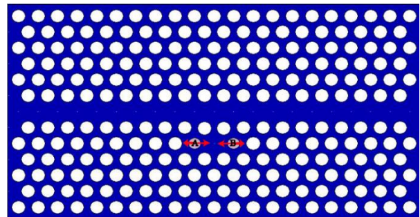
Şekil 6: Kaviteli FK yapısında A ve B ile gösterilen deliklerin yarıçaplarının değiştirilmesi veya içe veya dışa doğru kaydırılması.
