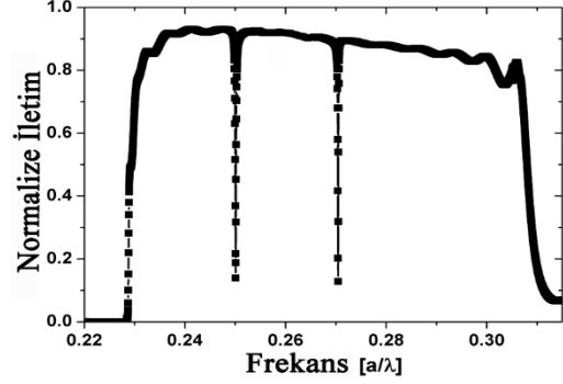
Şekil 4: Kaviteli fotonik kristal dalga kılavuzunun iletim spektrumu.
