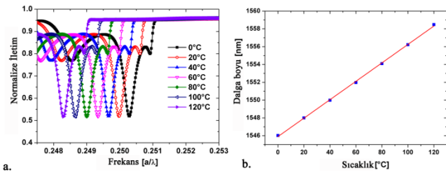
Şekil 12: Optimize edilmiş kavite yavaş ışık FKD yapısının sıcaklığa bağlı olarak kavite rezonans bandının değişimi. (b): Kavite rezonans merkez dalga boyunun sıcaklıkla değişimi.
