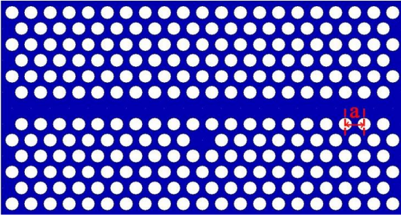
Şekil 1: Kaviteli FKD yapısı.
