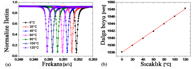
Şekil 9: Optimize edilmiş kaviteli FKD yapısının sıcaklığa bağlı olarak. (a): Kavite rezonans düşüş bandının değişimi. (b): Kavite rezonans merkez dalga boyunun sıcaklıkla değişimi.
