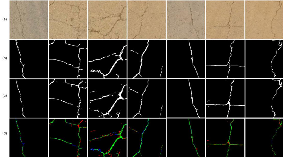
Şekil 6. Derin öğrenme tabanlı çatlak segmentasyonunun başarımları: (a) Gerçek görüntü, (b) Gerçek (etiketli) çatlak maskesi, (c) CT-CrackSeg tarafından tahmin edilen maskeler, (d) Kırmızı (Yanlış Pozitif), Mavi (Yanlış Negatif), Yeşil (Doğru Pozitif).
