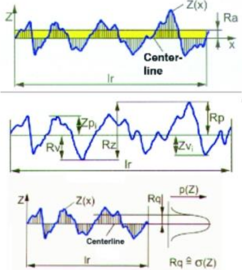
Şekil 2. Yüzey pürüzlülük profil örneği [34].
