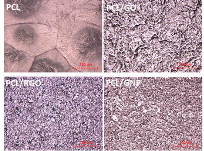
Şekil 5. Katkısız PCL ve filmlerin OM görüntüleri.
