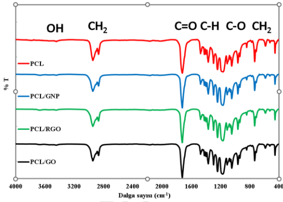
Şekil 4. Katkısız PCL ve filmlerin FTIR spektrumları. Figure 4. FTIR spectra of PCL and its films.
