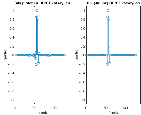
Şekil 6. LFM sinyalinin AKFD taban matrisi ile çözülmesi ve sıkıştırılmış hale getirilmesi Figure 6. Decoding the LFM Signal with the DFrFT Base matrix and compressing
