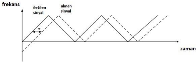
Şekil 1. İletilen ve yansıyan dalganın zaman-frekans gösterimi. Figure 1. Time-frequency presentation of transmitted and received signal.
