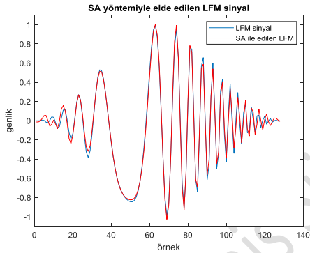
Şekil 8. SA yöntemiyle elde edilen LFM sinyal Figure 8. LFM Signal reconstructed by CS method.
