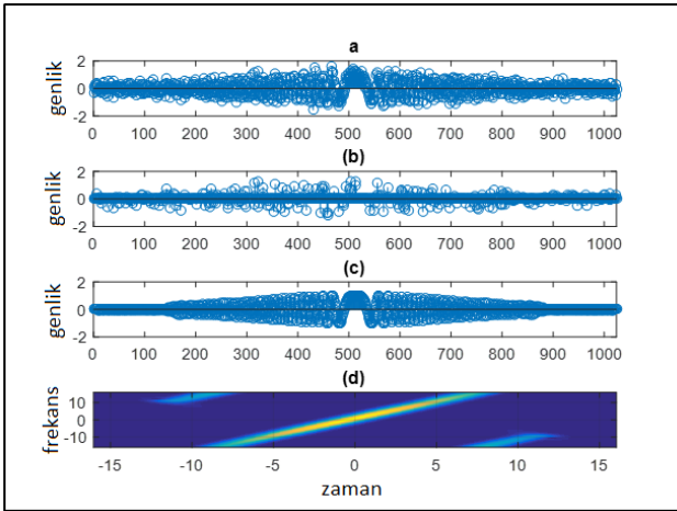
Şekil 13. (a) 1024 uzunluklu FMSDR sinyal, SNR=5dB (b) 256 uzunluklu rasgele FMSDR sinyal örneği alınmakta (c) Rasgele ölçümlerden elde edilen 1024 uzunluklu FMSDR sinyal (d) Geri elde edilen FMSDR sinyalin zaman-frekans düzlemi
