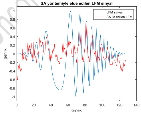
Şekil 11. Klasik FD taban matrisi kullanıldığında SA yöntemiyle elde edilen LFM sinyal
