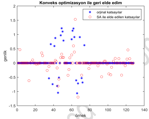
Şekil 10. Klasik FD taban matrisi kullanılarak rasgele ölçümlerden konveks optimizasyon sonucu geri çatım
