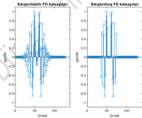
Şekil 9. LFM sinyalin klasik FD taban matrisi ile çözülmesi ve sıkıştırılmış hale getirilmesi
