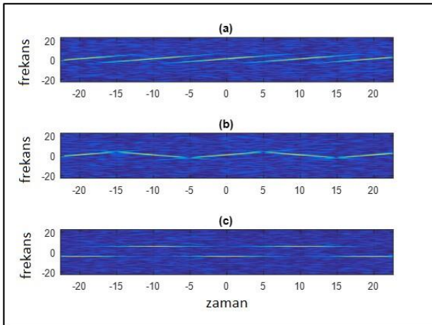
Şekil 2. Zaman-frekans düzleminde FMSDR sinyalleri için yaygın modülasyon modelleri a) testere dişi modülasyonlu, b) üçgen modülasyonlu, c) kare dalga modülasyonlu Figure 2. Common modulation patterns on time-frequency plane for FMCWR signals (a)sawtooth modulated (b) triangular modulated (c)square wave modulated.
