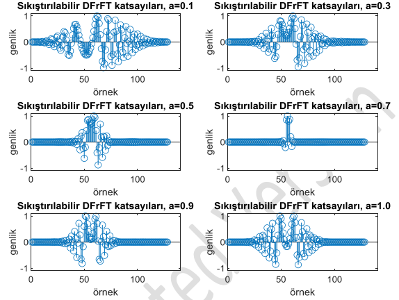
Şekil 5. LFM sinyalinin AKFD matrisi tabanındaki seyrek sıkıştırılabilir(seyrek) katsayıları Figure 5. Compressible(sparse) coefficients of the LFM signals analyzed by the DFrFT matrix
