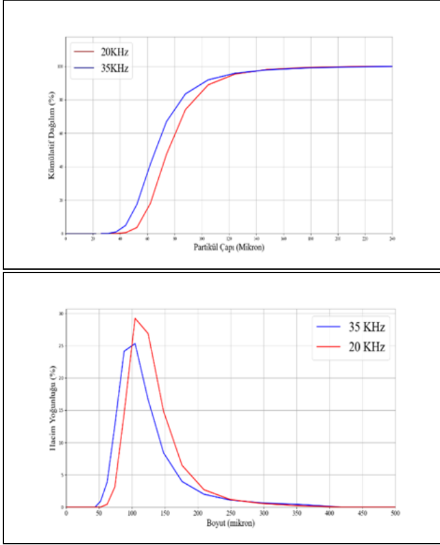
Şekil 2. Farklı frekanslarda üretilen tozların parçacık boyut dağılımı.
