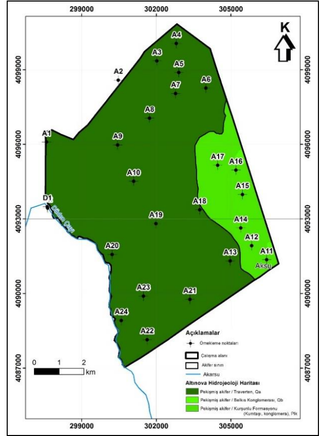
Şekil 5. Çalışma alanı hidrojeoloji haritası.
