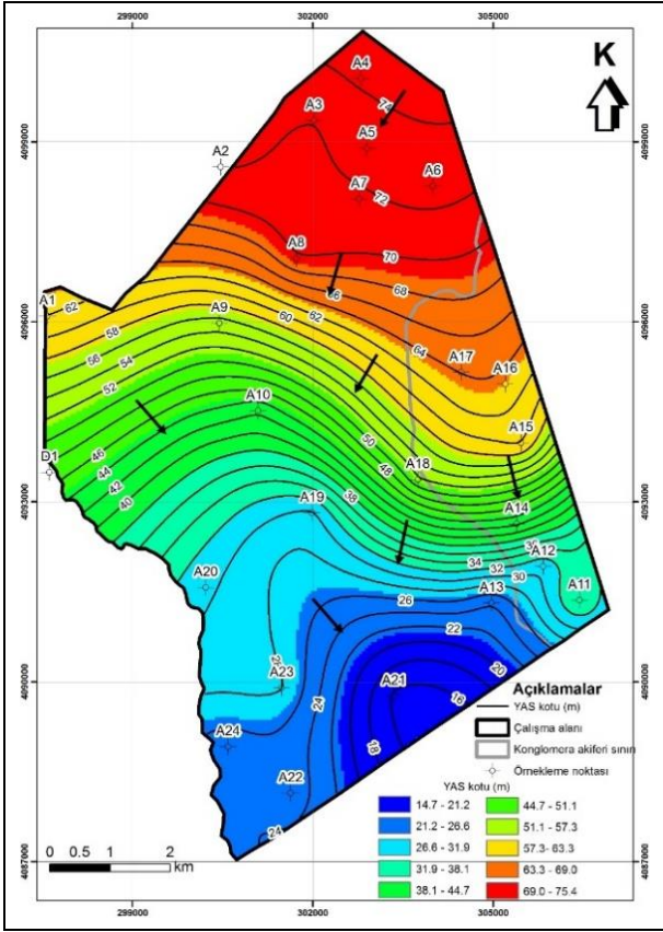
Şekil 6. Altınova akiferi yeraltısuyu kotu haritası(2015-Kasım).
