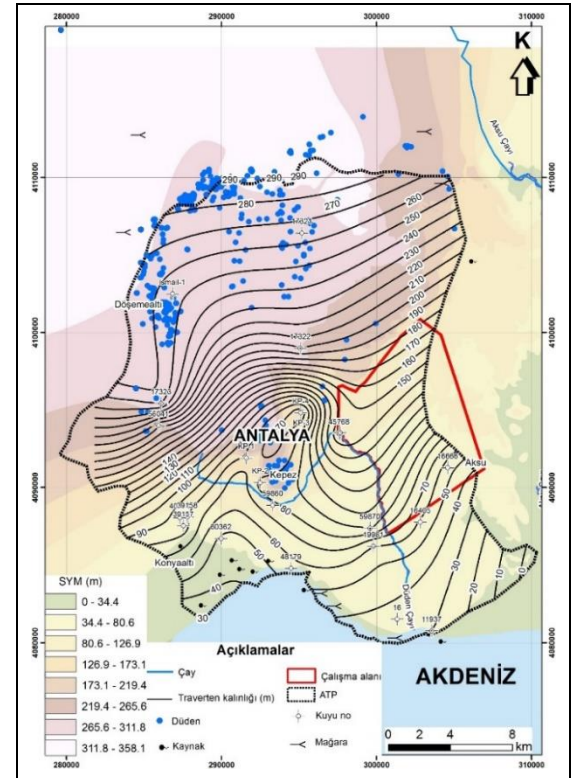
Şekil 2. ATP karst yapıları ve traverten kalınlık haritası.
