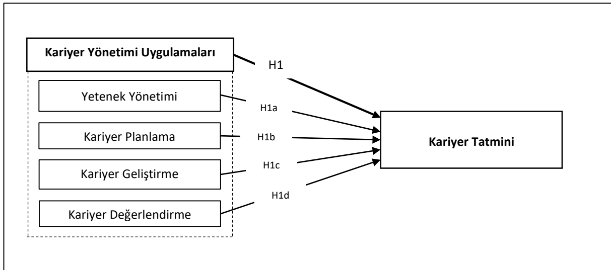
Şekil 1. Araştırma modeli
