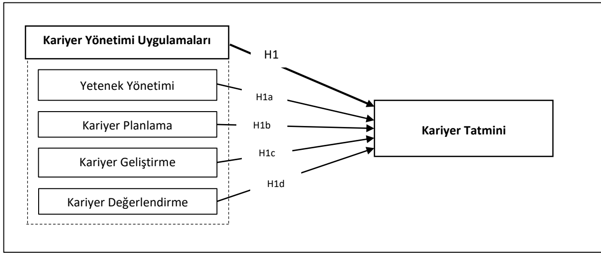
Şekil 1. Araştırma modeli
