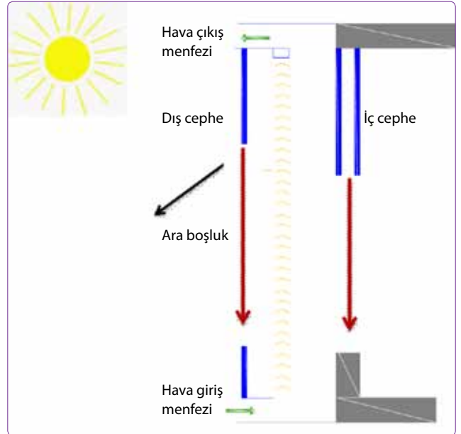
Şekil 1. Çift cidarlı cephe sistemi.
